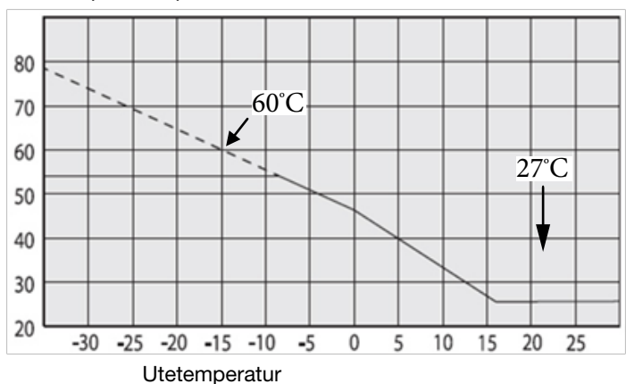
Primär panntemperatur
