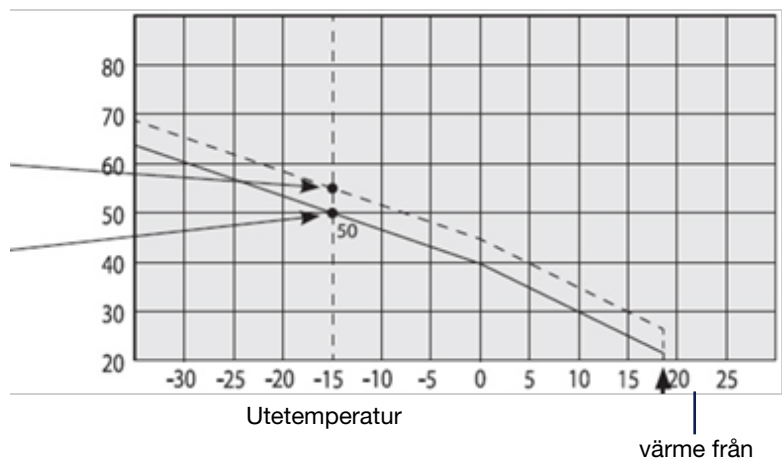
Primär panntemperatur
