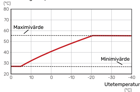
Framledningstemperatur
